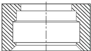
Perfil a maquinar por interpolación Interpolated machining profile
